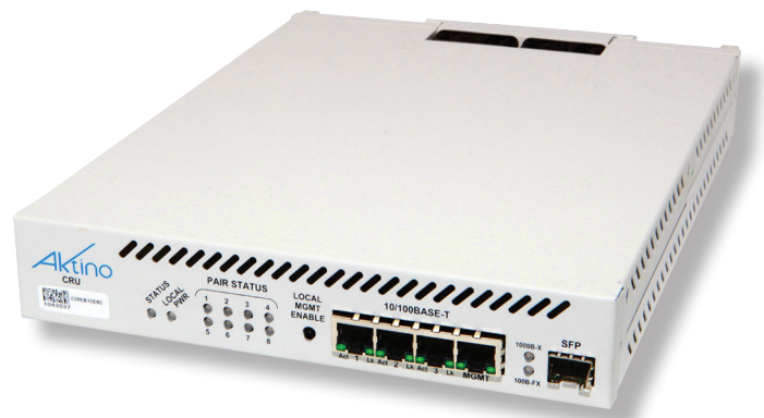
Positron Aktino AK500 Compact Unit
